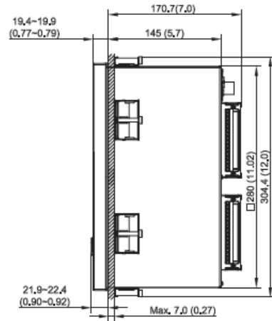
側面圖
