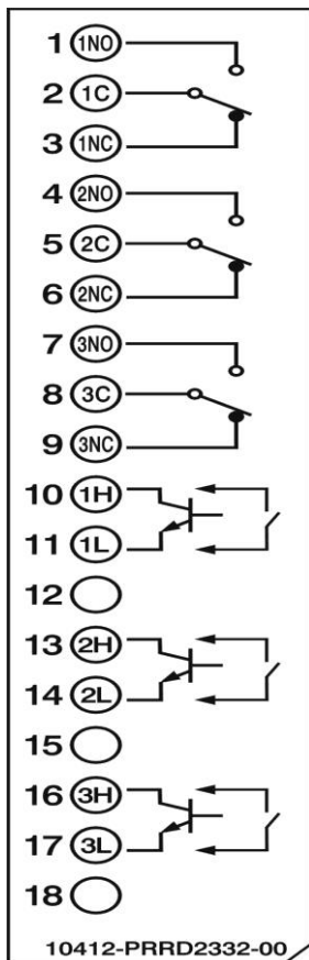
RD233 繼電器輸出和數位輸入卡接線端子圖
