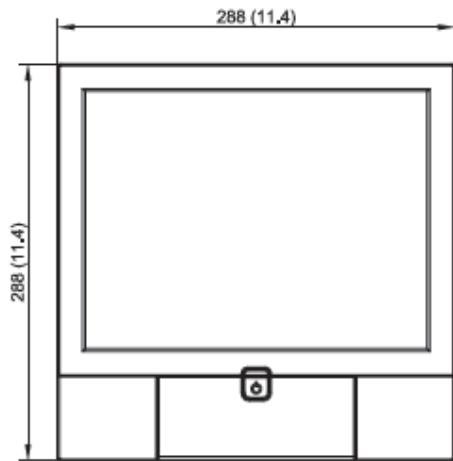
正面圖
