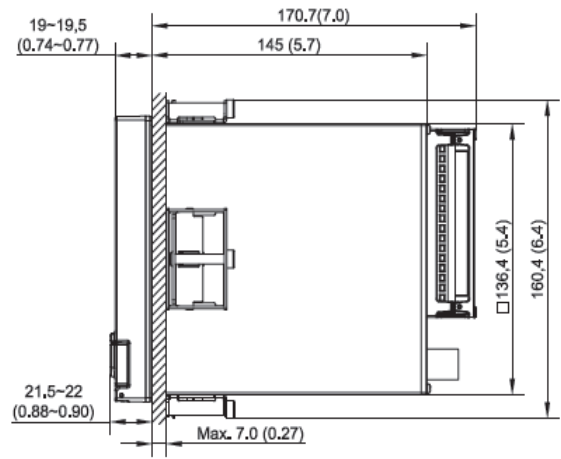
側面圖
