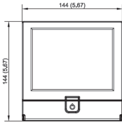
正面圖
