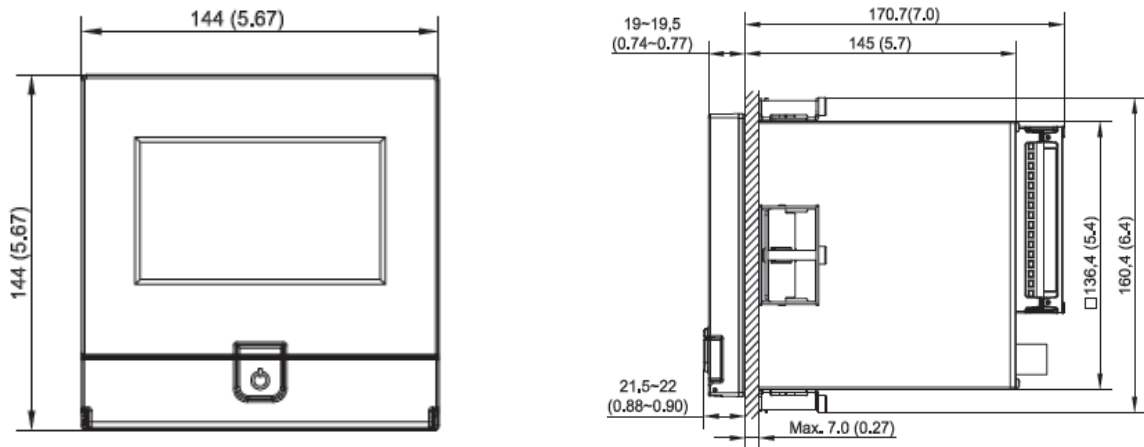
側面圖
