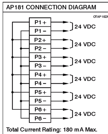
圖 2-23 24VDC 輔助電源卡(AP181)接線示意圖
