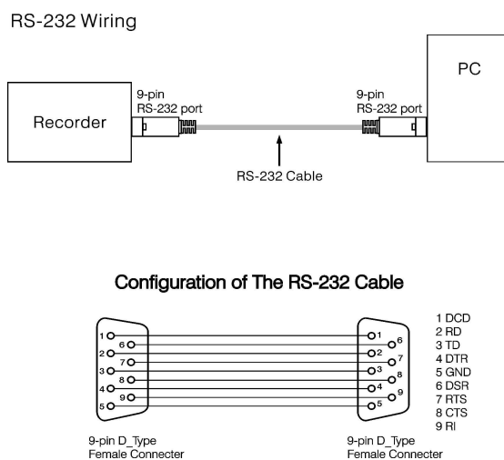
圖 2-24 RS232 接線示意圖
