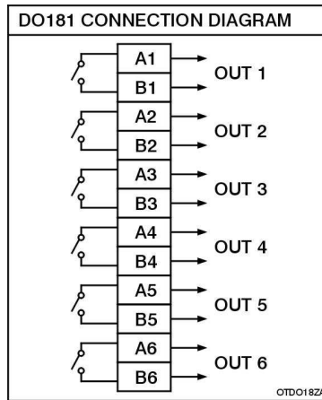
圖 2-20 數位輸出卡 (DO181) 接線示意圖
