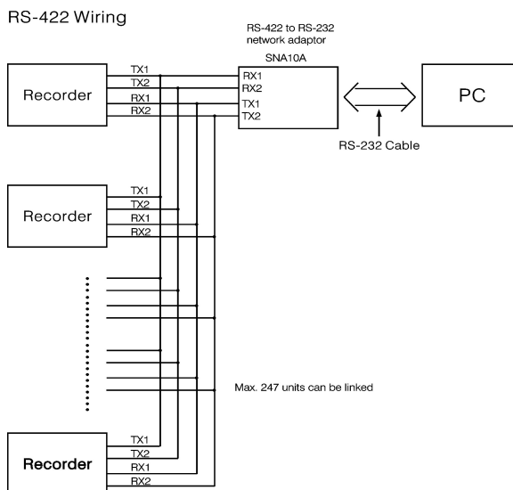
圖 2-25 RS422 接線示意圖
