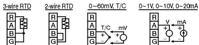
圖 2-18 類比輸入卡 (AI181/182/183) 接線示意圖
