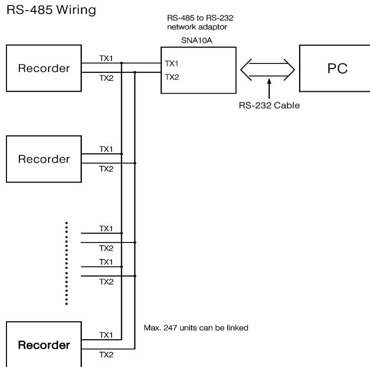
圖 2-26 RS485 接線示意圖
