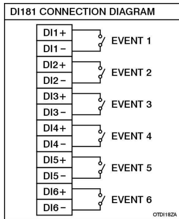
圖 2-21 數位輸入卡 (DI181) 接線示意圖
