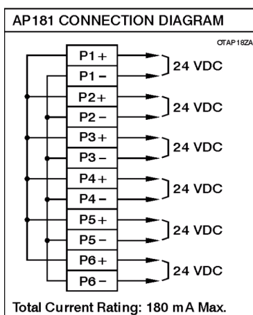
圖 2-23 24VDC 輔助電源卡(AP181)接線示意圖
