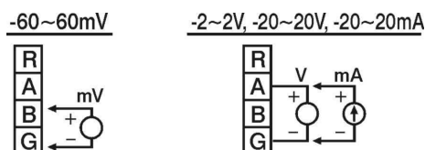
圖 2-19 電壓輸入卡 (AI181V/182V/183V) 接線示意圖
