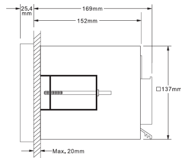
圖 2-2 側面圖
