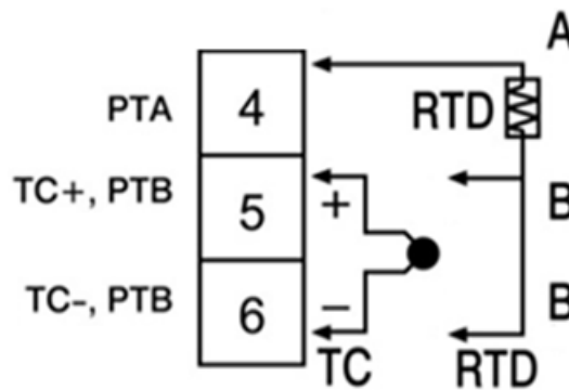
傳感器配線
