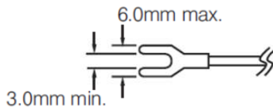
導線端子
