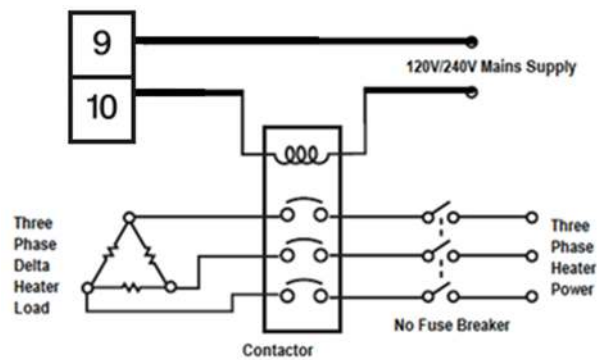
OP1 繼電器驅動接觸器
