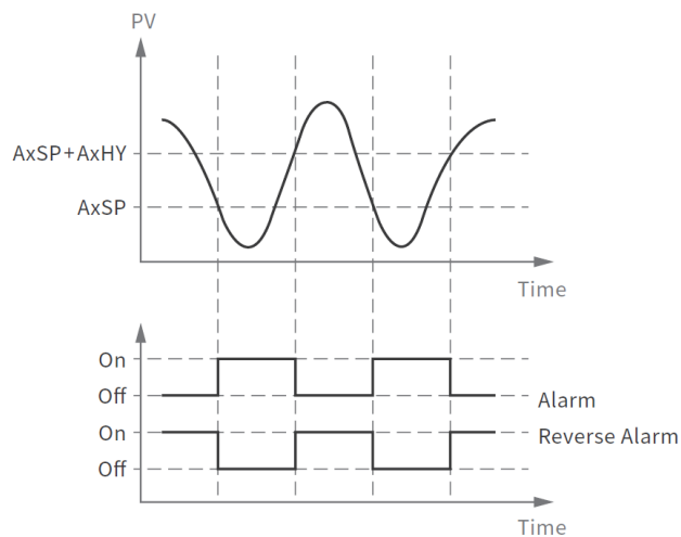
PV 低限警報 (PV.Lo)
