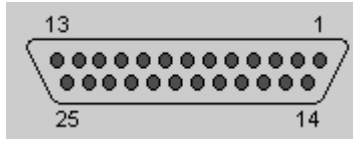
Fig: DB25 母
