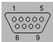
Fig: DB9 公
