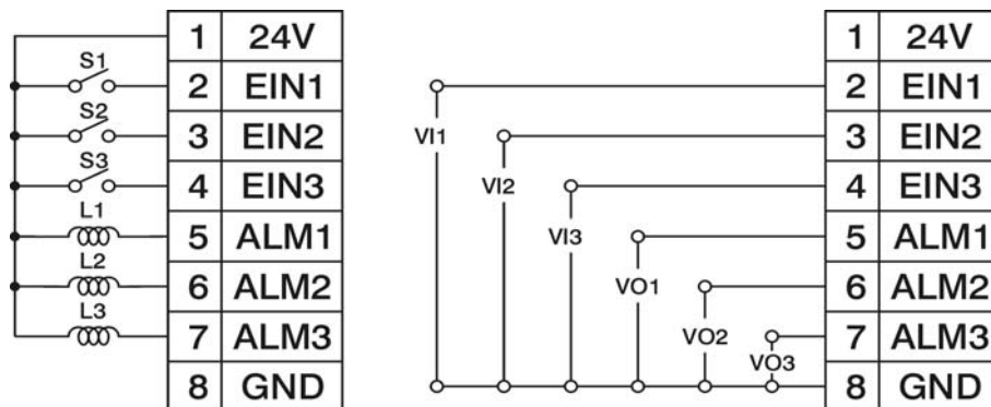
Fig: 接線說明
