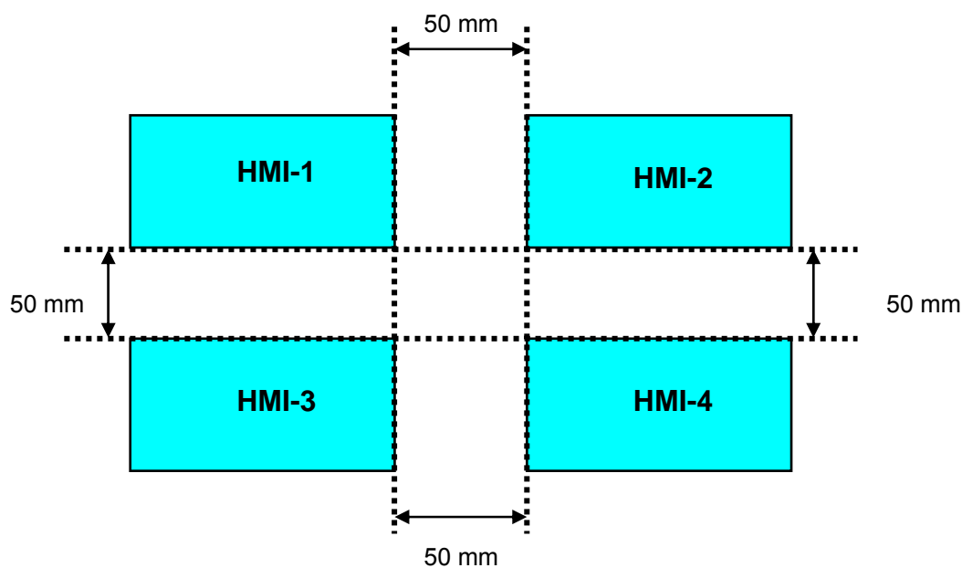
Fig: HMI 安裝空間
